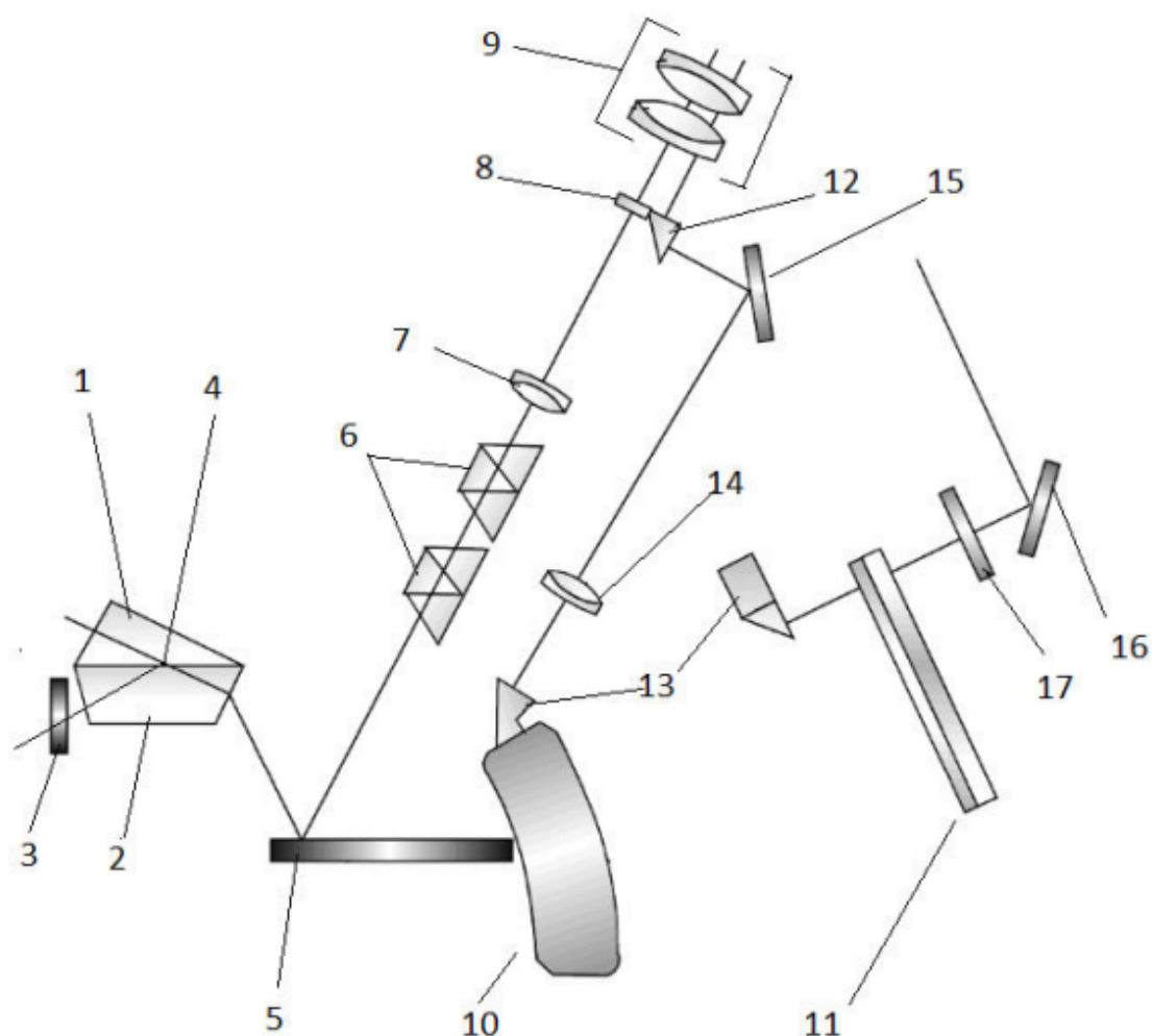
Рисунок 1 - Схема оптическая рефрактометра
