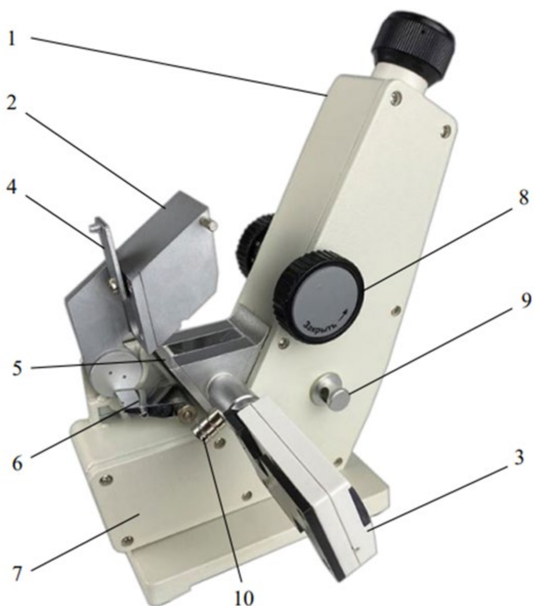
Рисунок 3 – Вид рефрактометра с левой стороны
