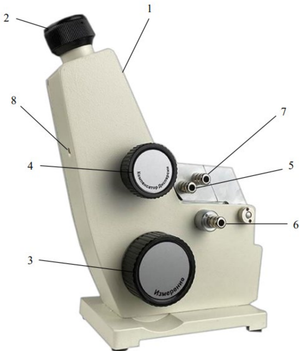
Рисунок 2 – Вид рефрактометра с правой стороны
